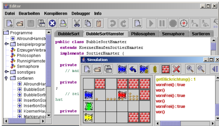
Abbildung 2: Der Hamster-Simulator
